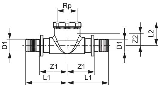
TECEflex, трійник, внутрішня різьба
