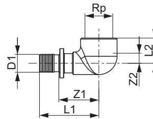
TECEflex компактний кутовий фітинг, червона латунь/кремнієва бронза
