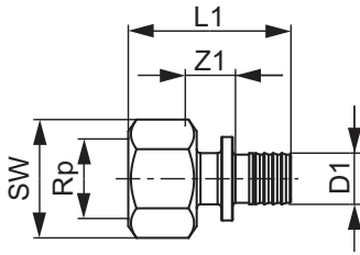
TECEflex, перехідник із внутрішньою різьбою
