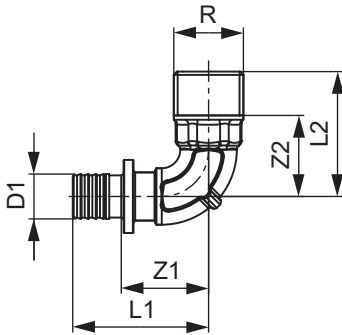
TECEflex, кутник із зовнішньою різьбою
