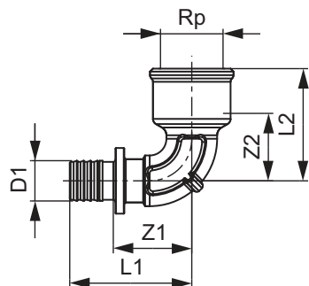
TECEflex, кутник із внутрішньою різьбою
