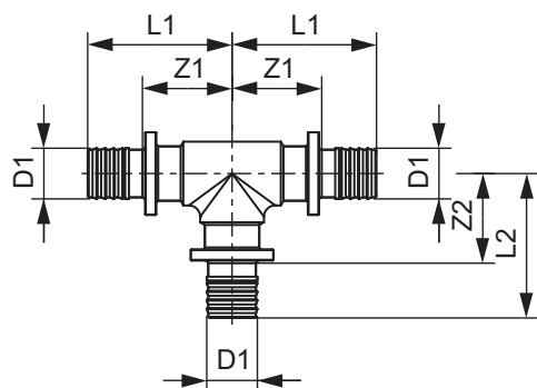
TECEflex, трійник
