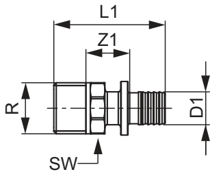
TECEflex, перехідник із зовнішньою різьбою
