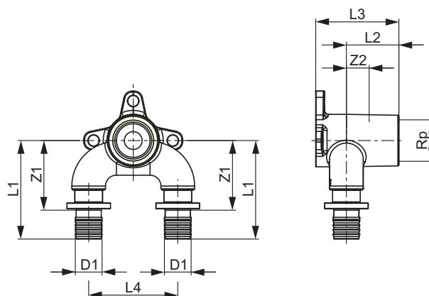
TECEflex, двовивідний настіінний кутник, незначні втрати тиску, червона латунь/кремнієва бронза
