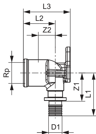
TECEflex, настіінний кутник
