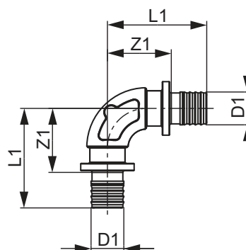
TECEflex, кутник 90°, незначні втрати тиску, червона латунь/кремнієва бронза
