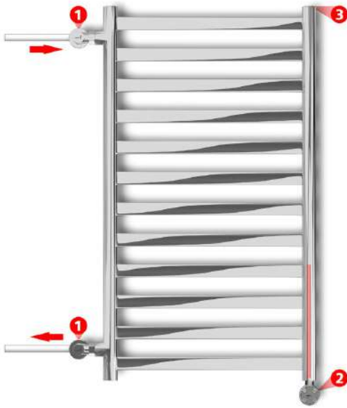
Комбіноване бічне підключення
