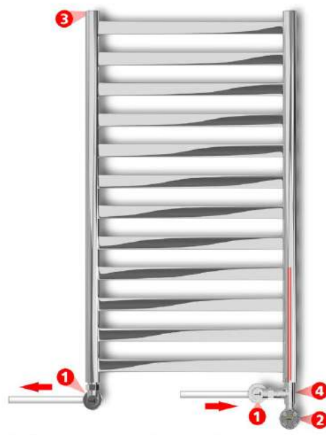
Комбіноване підключення з трійником
