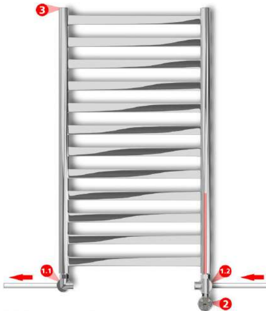
Комбіноване підключення через кран під ТЕН
