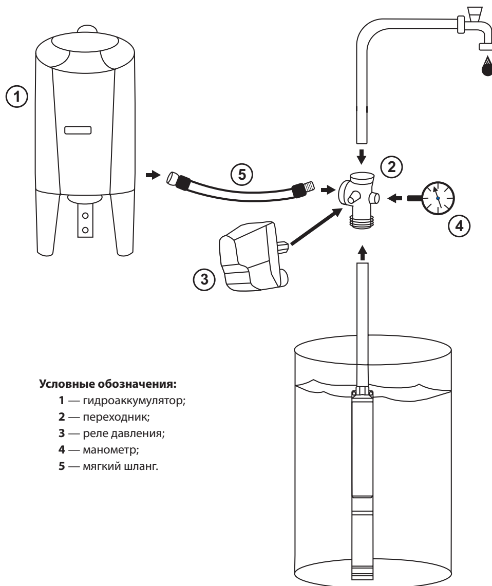
Система водоснабжения с использованием скважинного электронасоса
